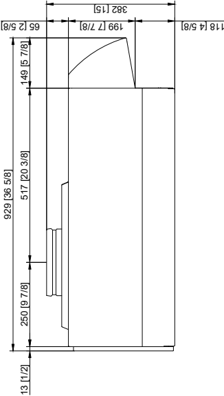
Seitenansicht Side view Vue de côté
