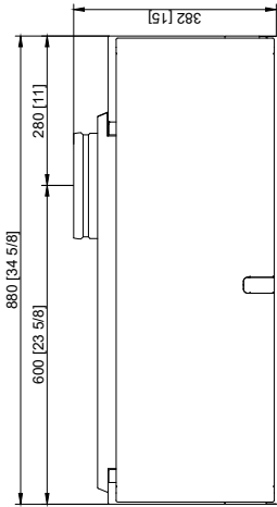
Rückansicht Back view Vue arrière
