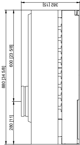
Vorderansicht Front view Vue de face
