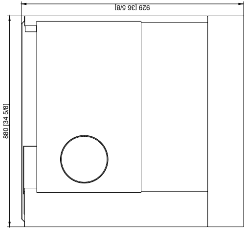
Draufsicht Top view Vue de dessus
