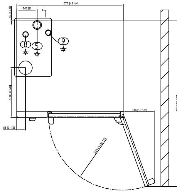
Mindestabstand bei Wandaufstellung (rechts) Minimum distance for wall installation (right) Distance minimale pour l'installation murale (droite)
