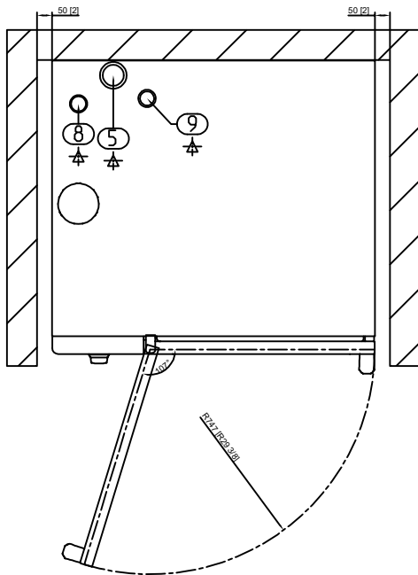
Abstandsmaße für Nischenaufstellung (gelfen für Linksanschlag und Rechtsanschlag) Distance dimensions for niche installation (Apply to left hinged door and right hinged door) Dimensions d'écartement pour l'installation en niche (Valable pour butée gauche et butée droite)
