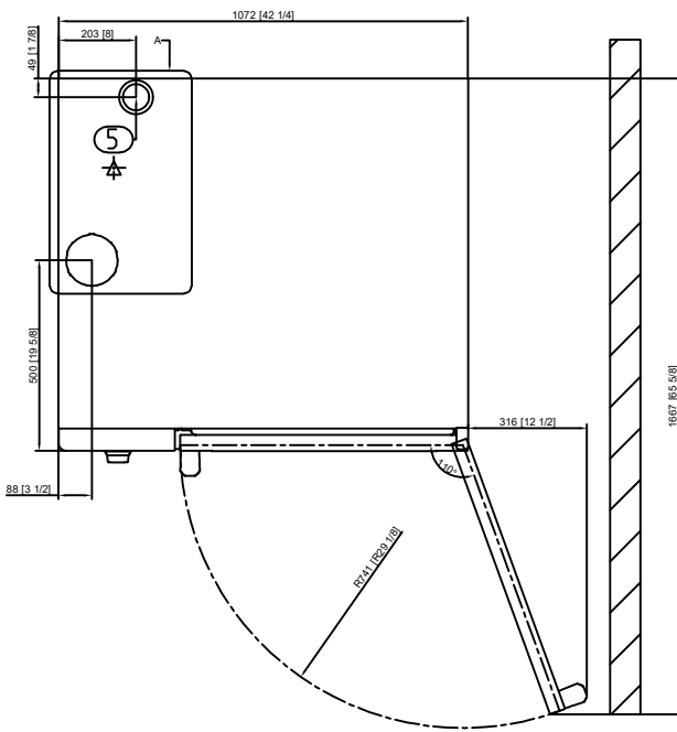
Mindestabstand bei Wandaufstellung (rechts) Minimum distance for wall installation (right) Distance minimale pour l'installation murale (droite)
