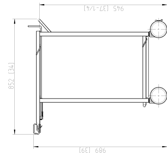
Seitenansicht side view
