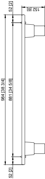
Seitenansicht mit Standard Füßen Side view with standard feet Vue de côté avec pieds standards
