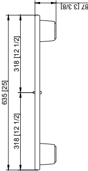
Seitenansicht mit niedrigen Füßen Side view with short feet Vue de côté avec pieds bas
