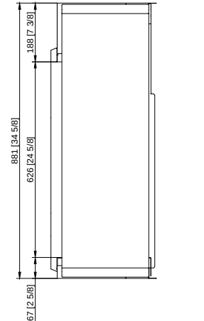
Rückansicht Back view Vue arrière
