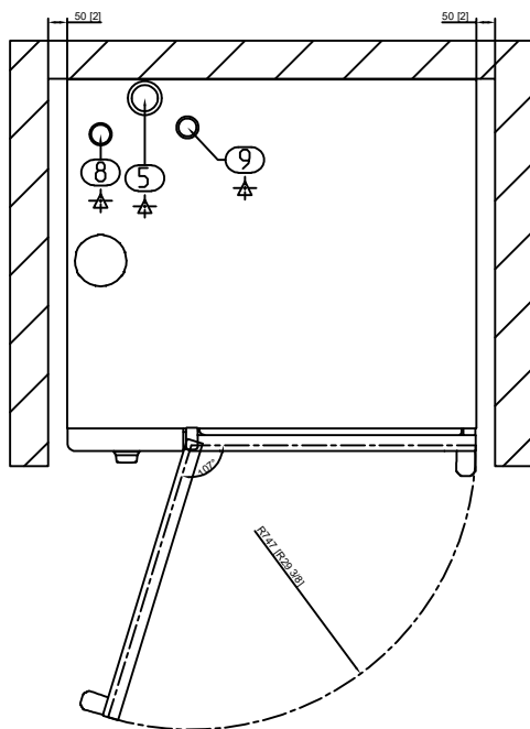
Abstandsmaße für Nischenaufstellung (gelten für Linksanschlag und Rechtsanschlag) Distance dimensions for niche installation (Apply to left hinged door and right hinged door) Dimensions d'écartement pour l'installation en niche (Valable pour butée gauche et butée droite)
