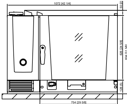
Rechtsanschlag Right hinged door Butée à droite
