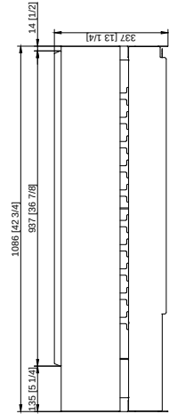
Vorderansicht Front view Vue de face
