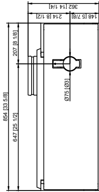
Rückansicht Back view Vue arrière
