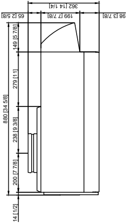
Seitenansicht Side view Vue de côté
